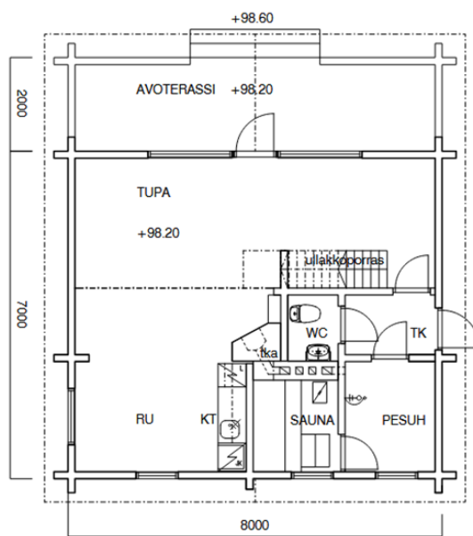
LOMARAKENNUS POHJAPIIRUSTUS 1 : 100
