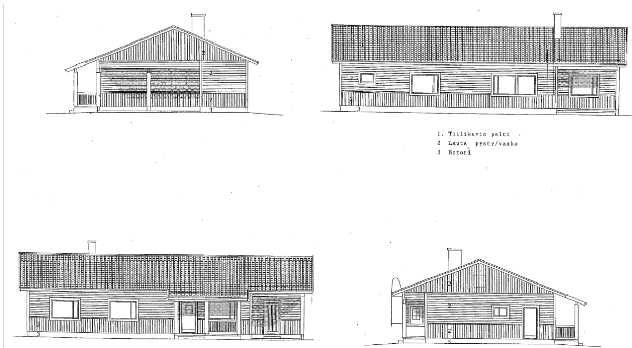
Julkisivut
