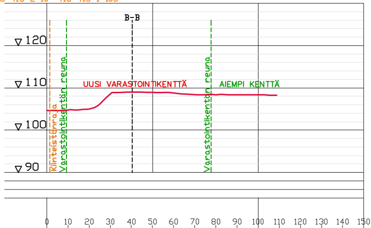
Leikkaus A-A
