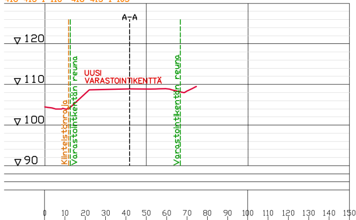
Leikkaus B-B
