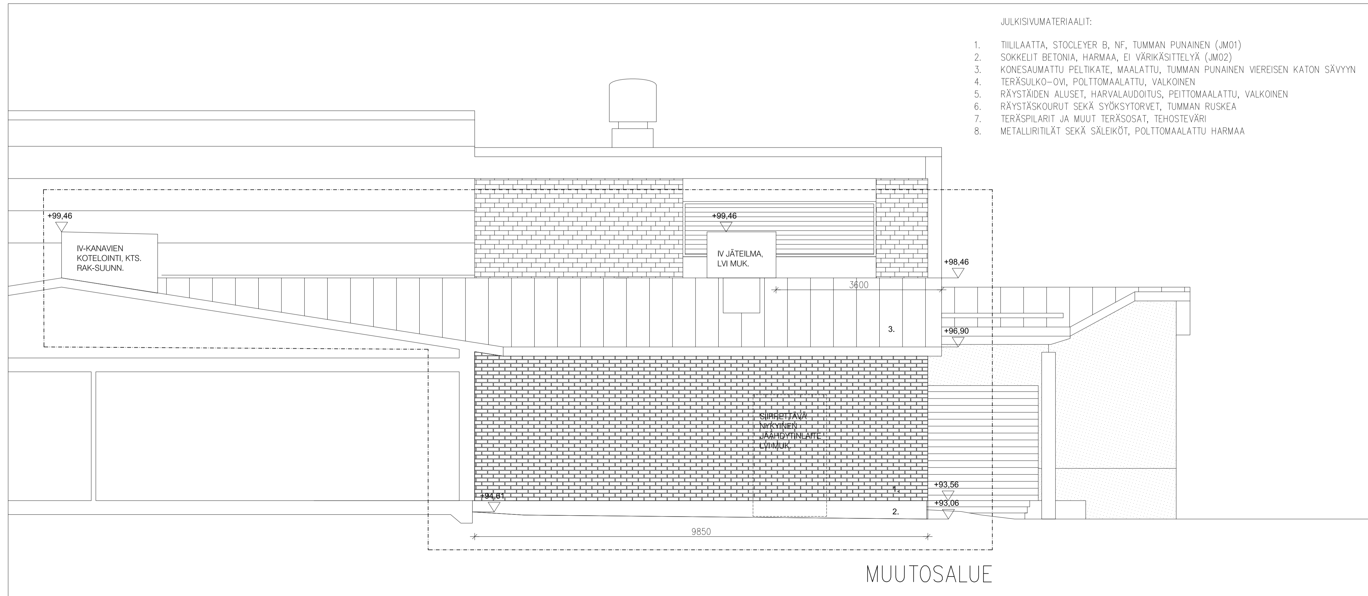
JULKISIVU ITÄÄN
